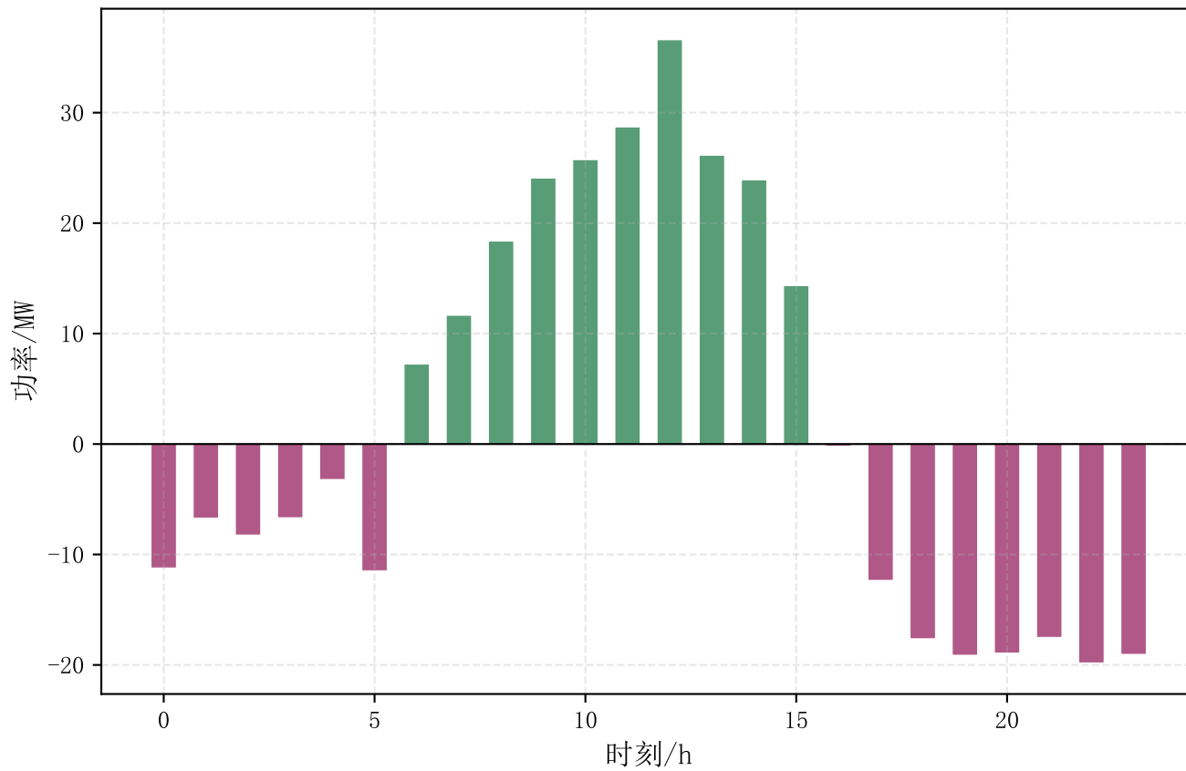
净负荷(正=余电上网, 负=购电)
