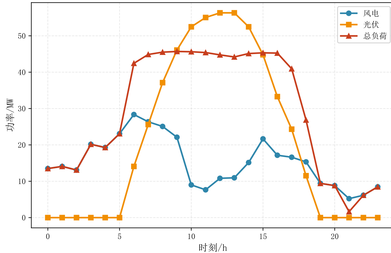
制氢功率跟随可再生出力
