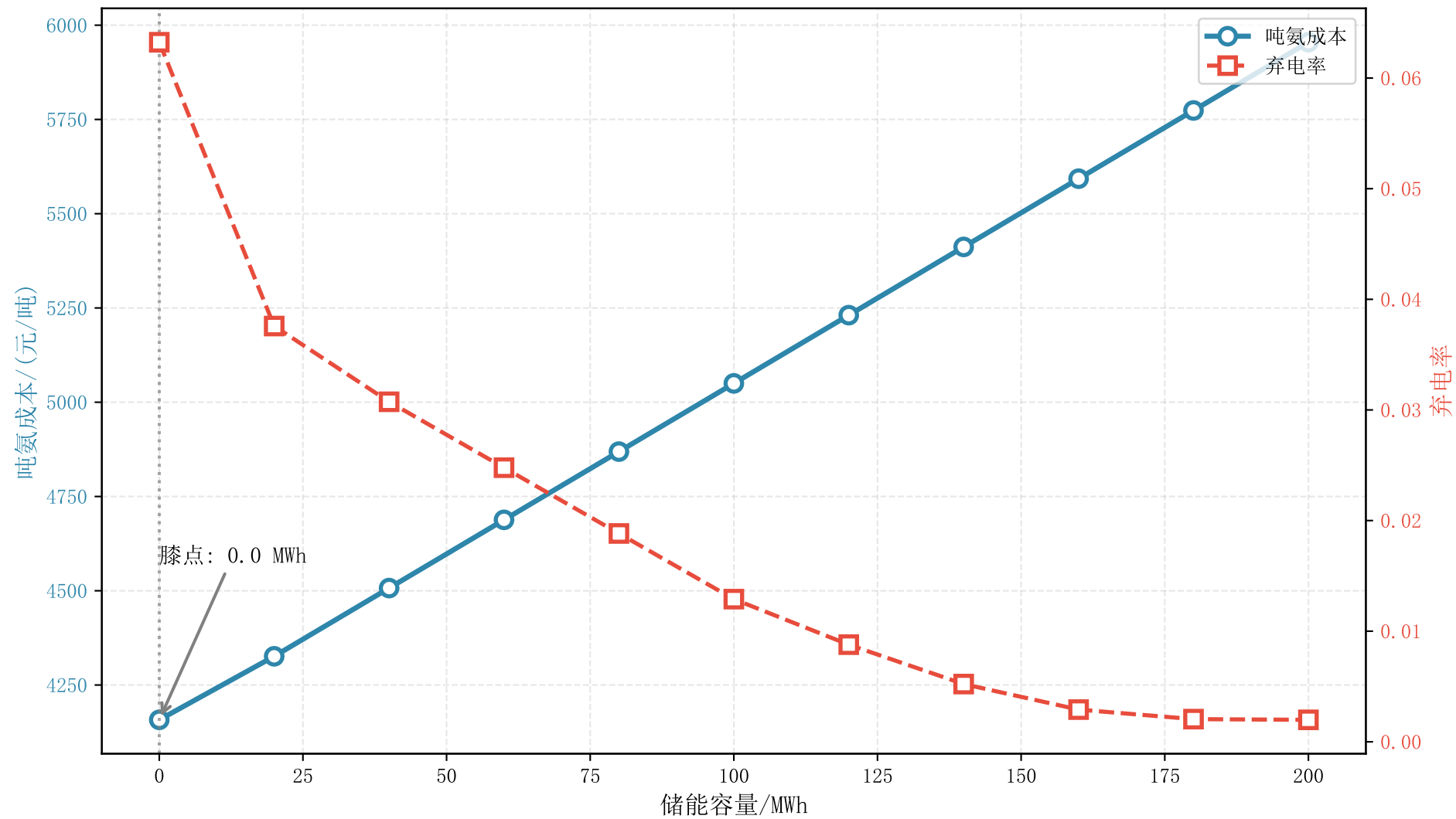
储能容量优化Pareto曲线
