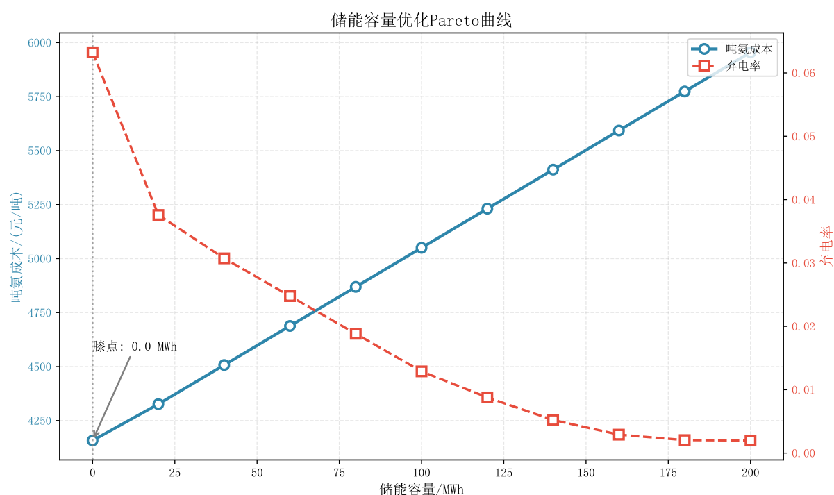
图 12 储能容量优化 Pareto 曲线
