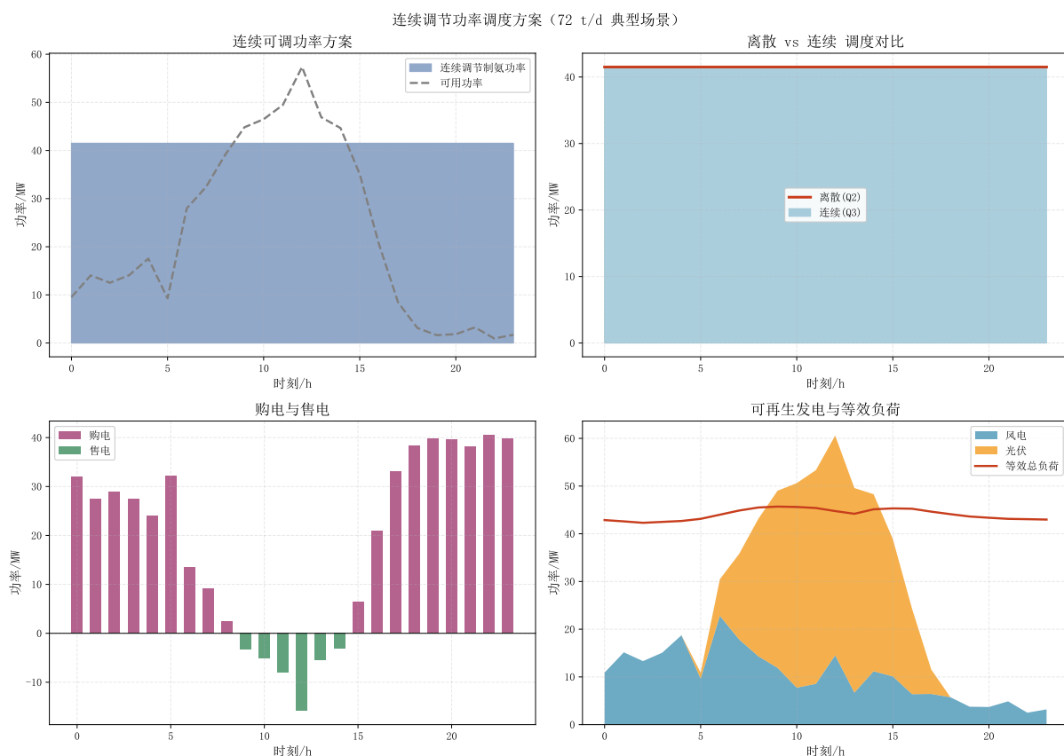
图 7 连续调节功率调度方案 (72 t/d 典型场景)
