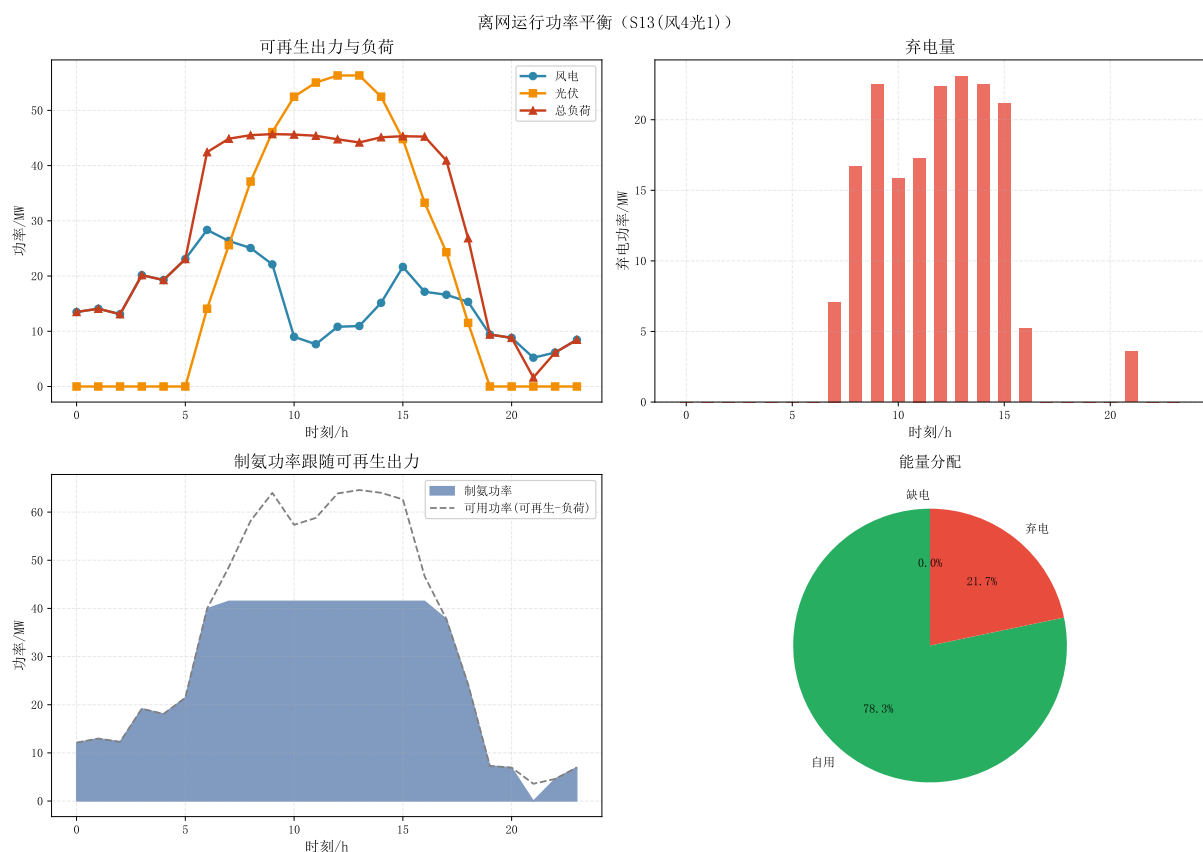
图 10 最大弃电场景 (S13 风 4 光 1) 离网运行功率平衡
