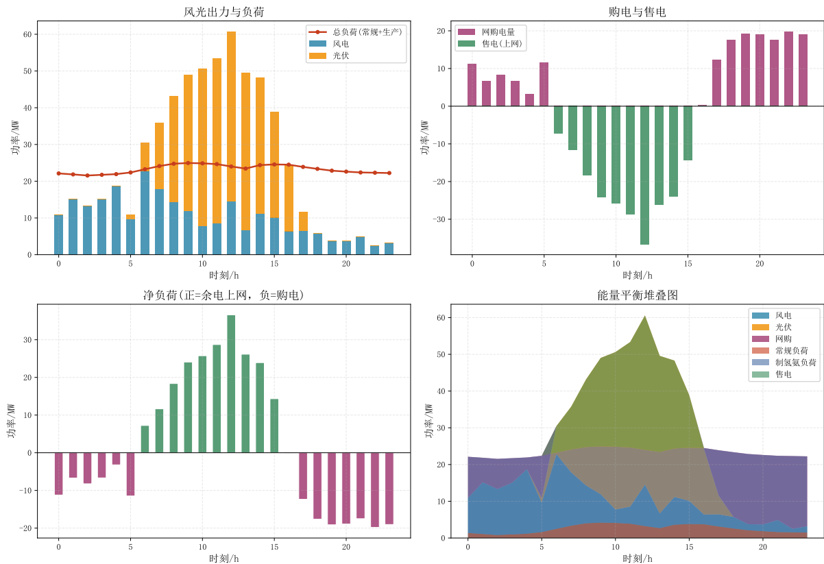
图 1 园区典型日功率平衡曲线
