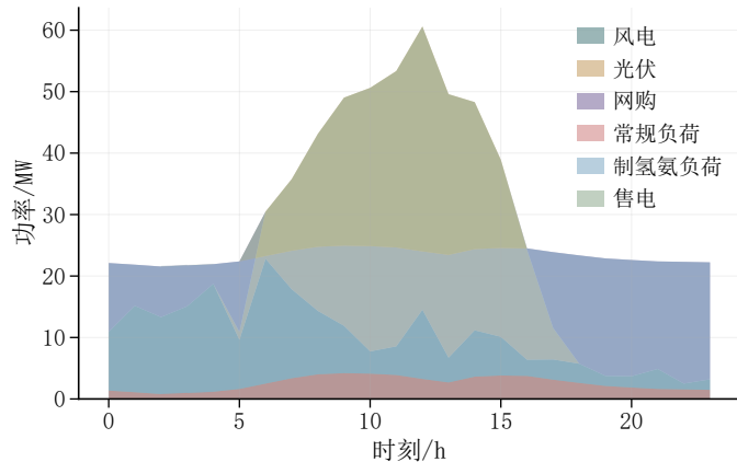
能量平衡堆叠图
