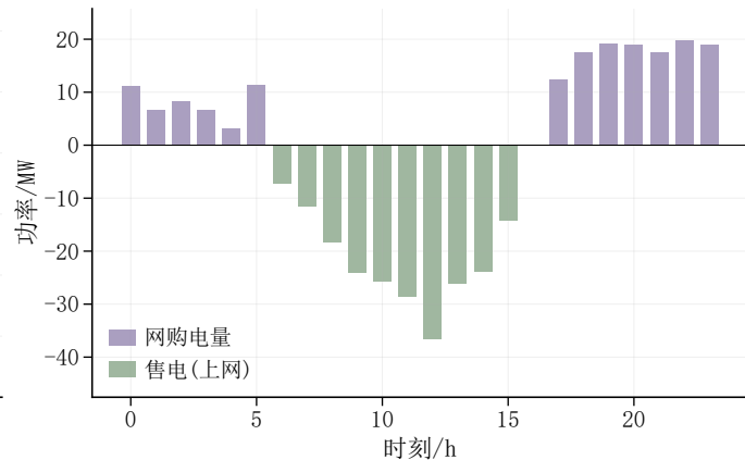
能量平衡堆叠图
