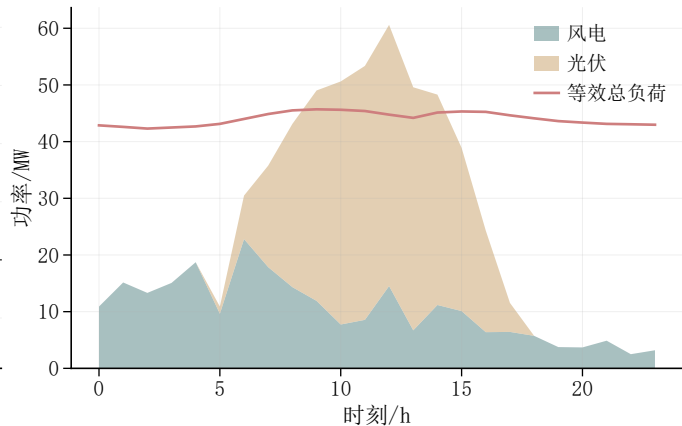
可再生发电与等效负荷
