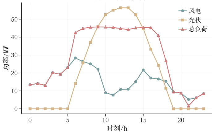
制氢功率跟随可再生出力
