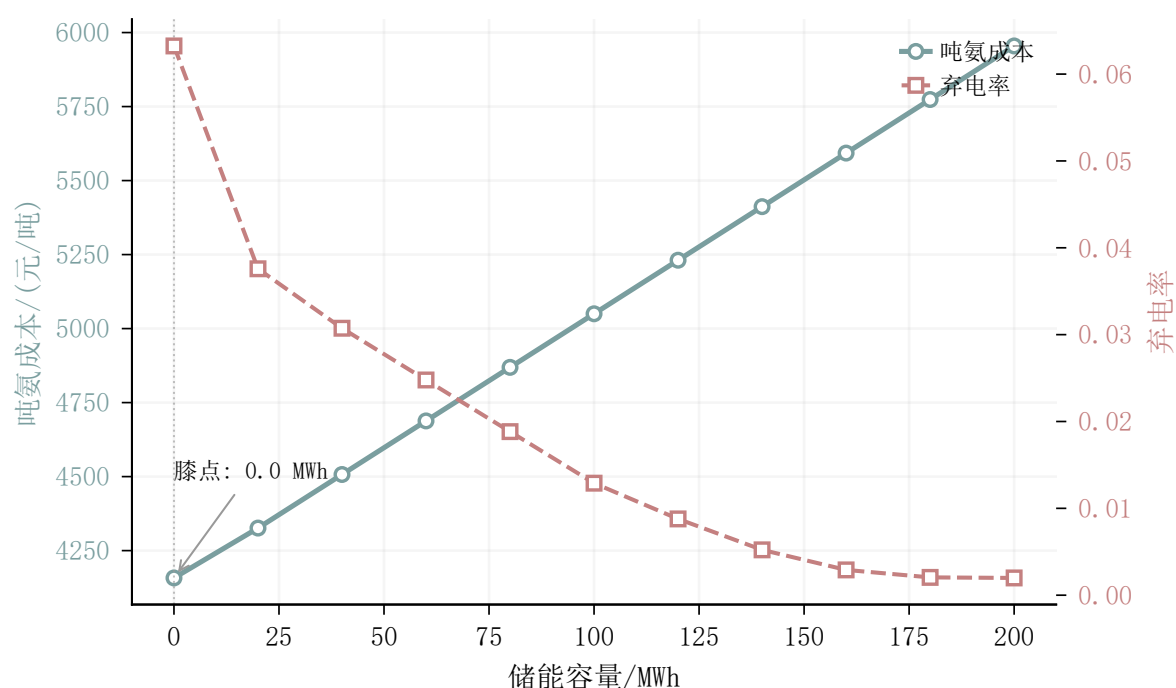
图 12 储能容量优化 Pareto 曲线
