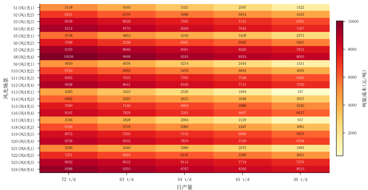
图 5 24 场景 × 5 产量吨氨成本热力图
