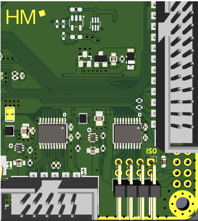
Figure 5: ISO/IEC 7816 Interface Sektion auf der Platine
