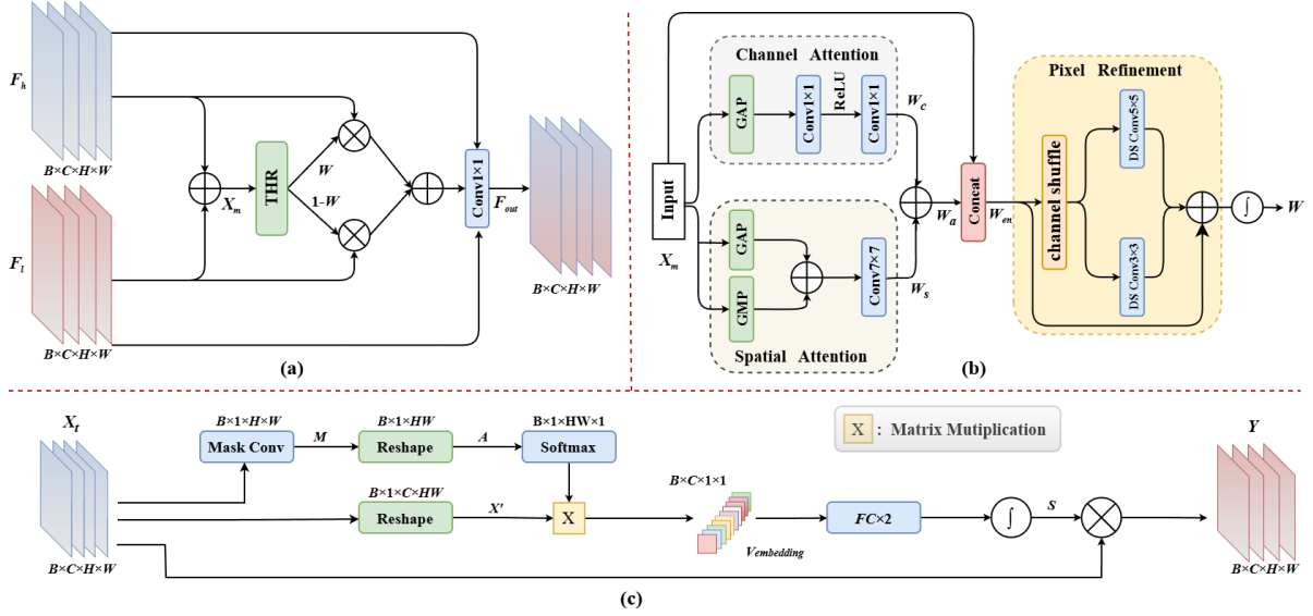
图 4.4 (a) 三级上下文融合模块(TCF) (b) 三重注意力层级精炼模块(THR) (c) 选择性嵌入分割头(SSH)
