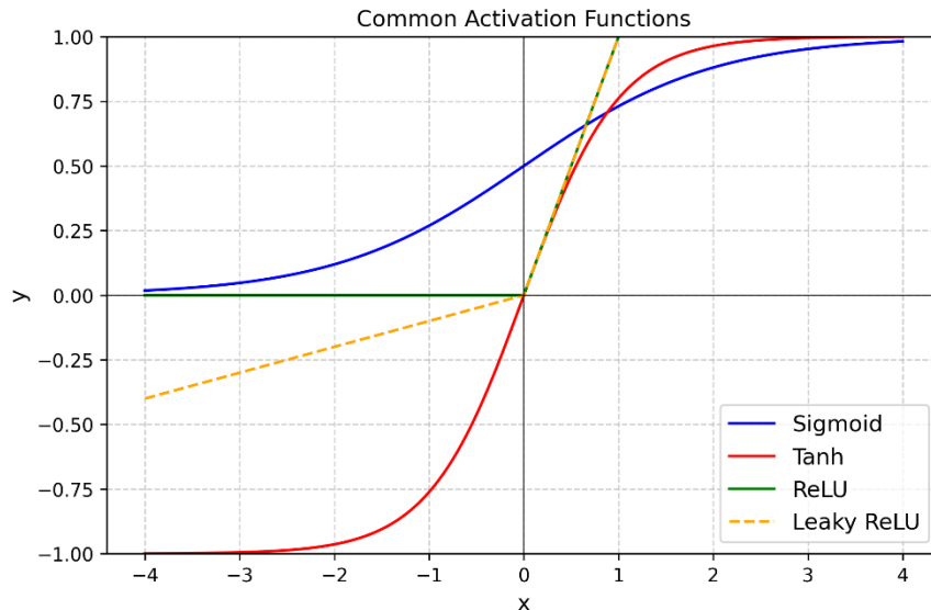
图 2.5 激活函数曲线图
