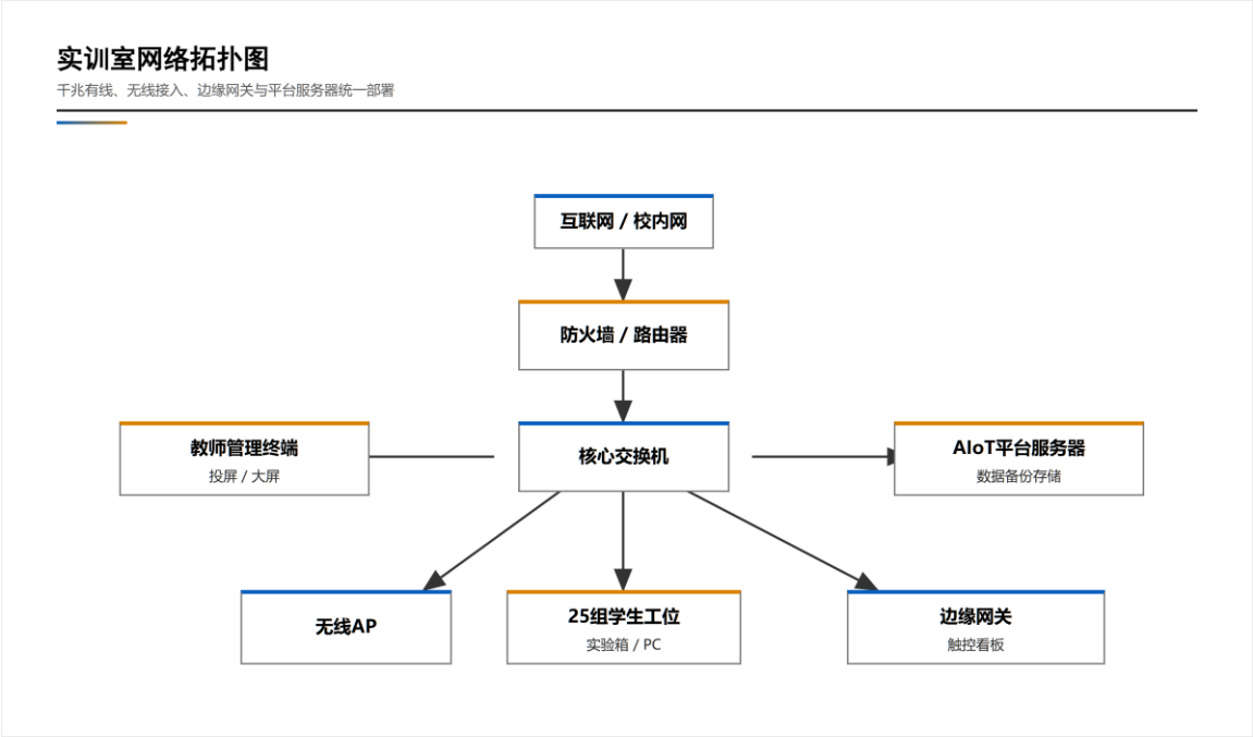
图 3-2 实训室网络拓扑图
