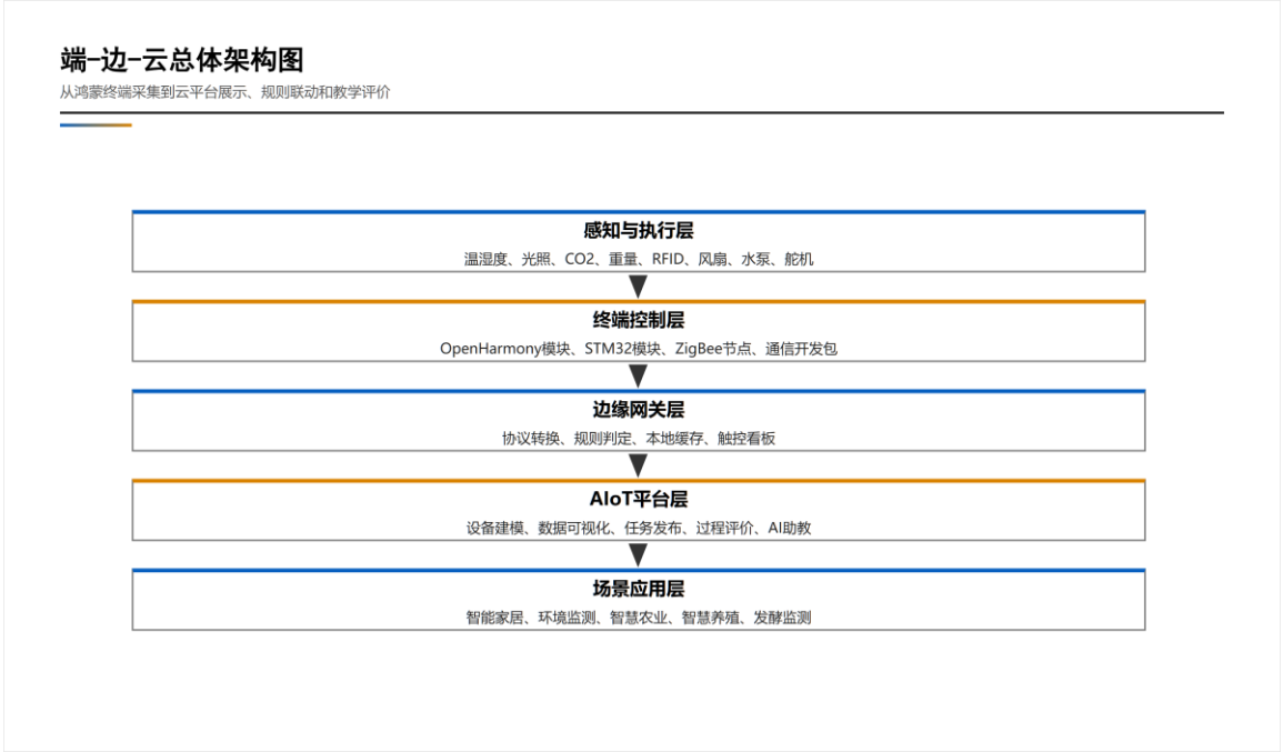
图 3-3 端-边-云总体架构图
