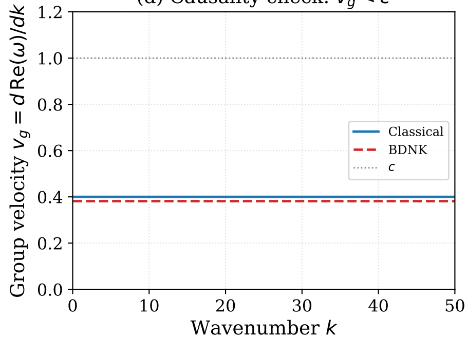
(d) Causality check: v_g < c
