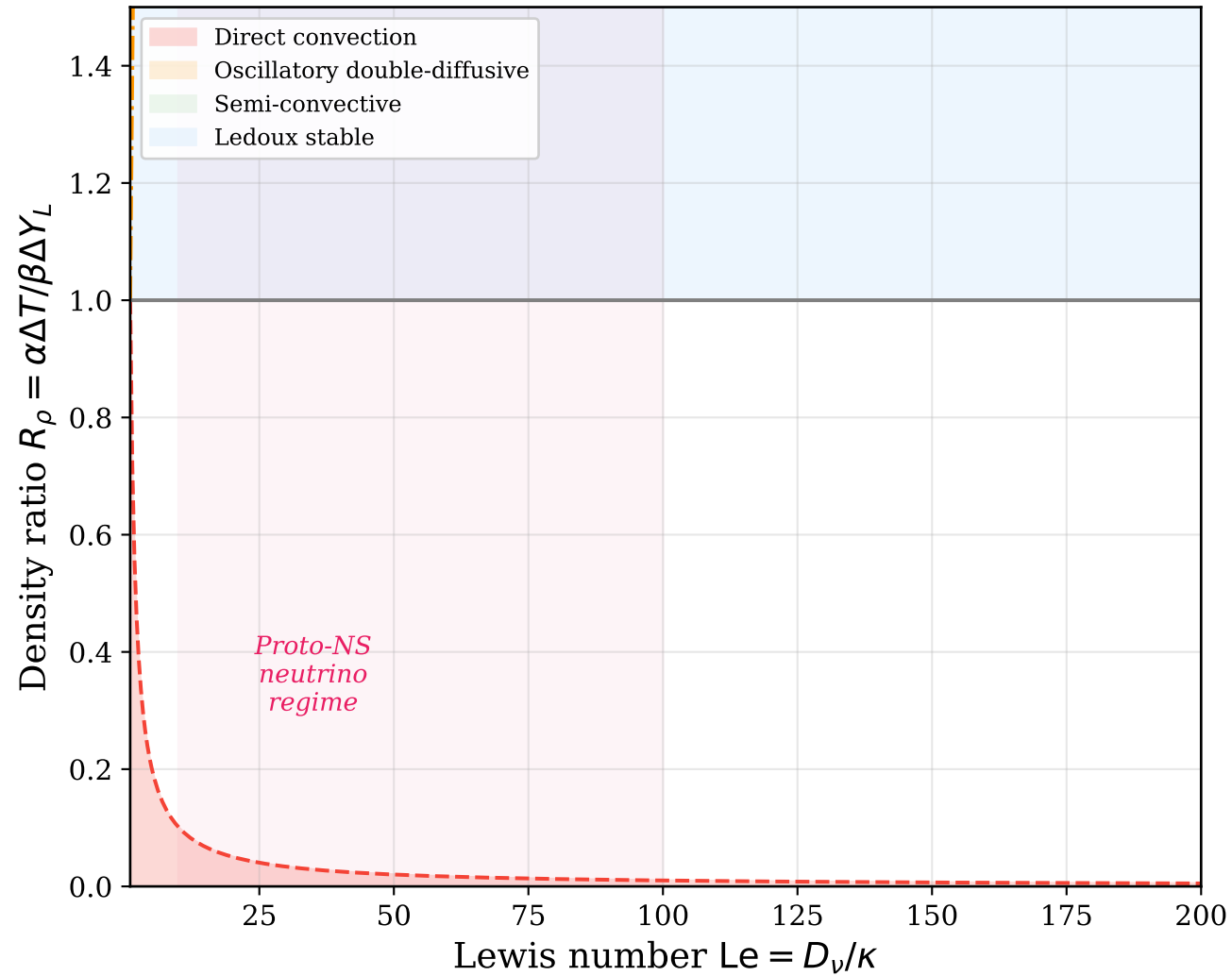
(a) Double-diffusive parameter space
