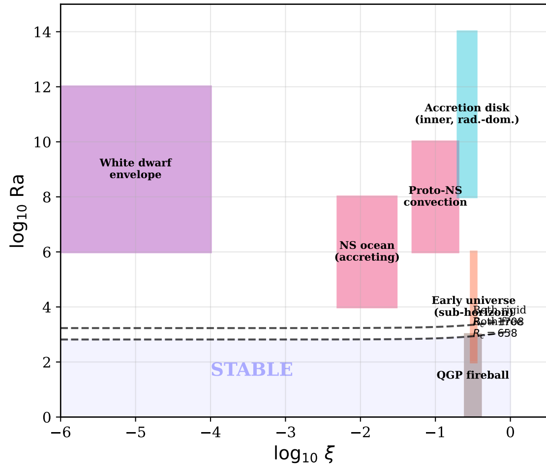
(a) Astrophysical parameter space
