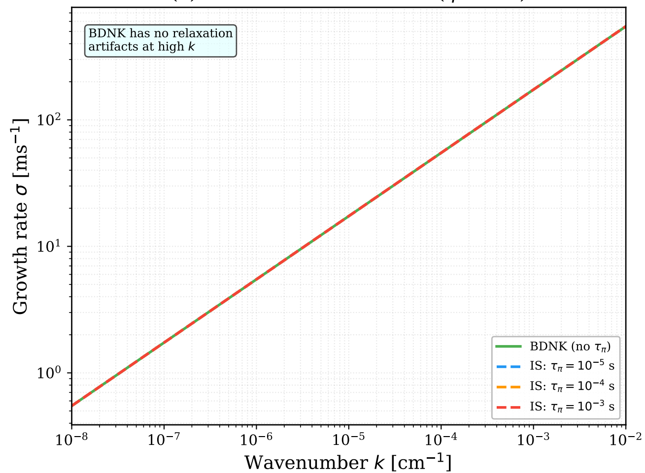
(d) BDNK vs Israel--Stewart ( \eta = 10^{17} )
