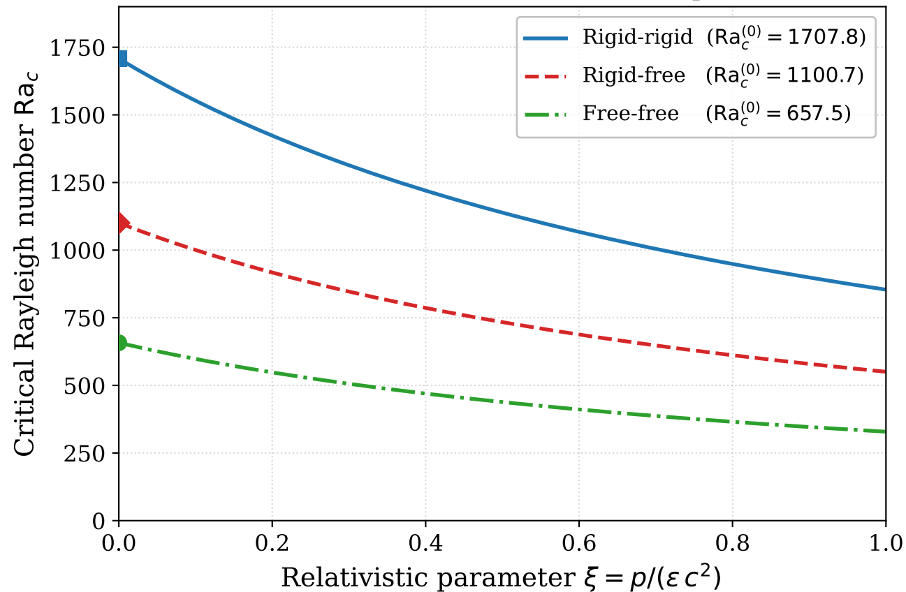
Bénard convection: Ra_c vs relativistic parameter
