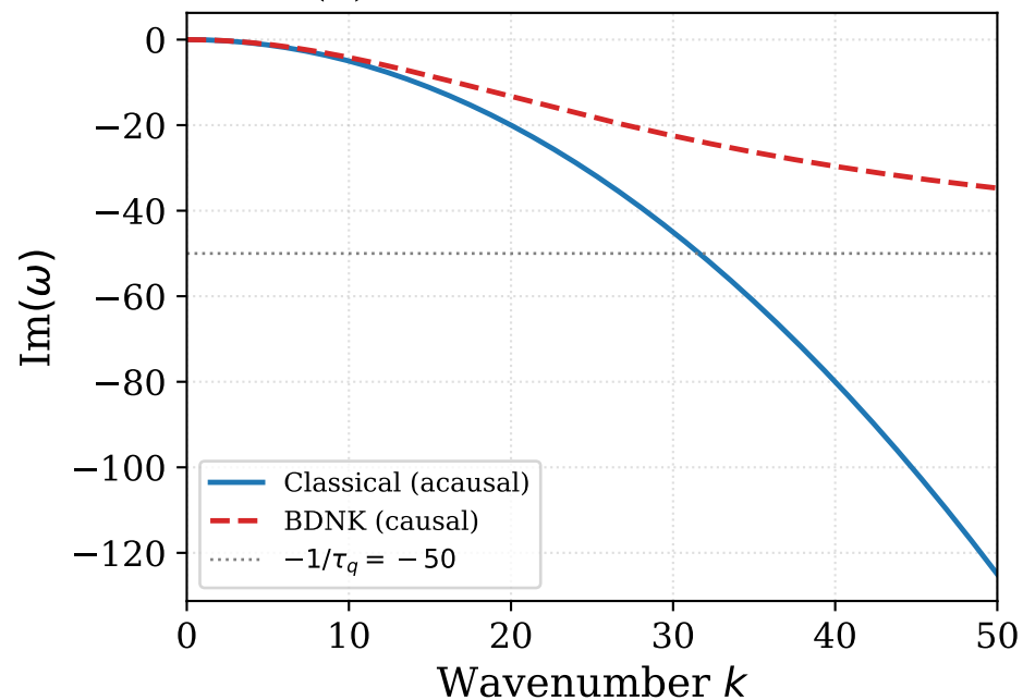
(b) Thermal diffusion mode
