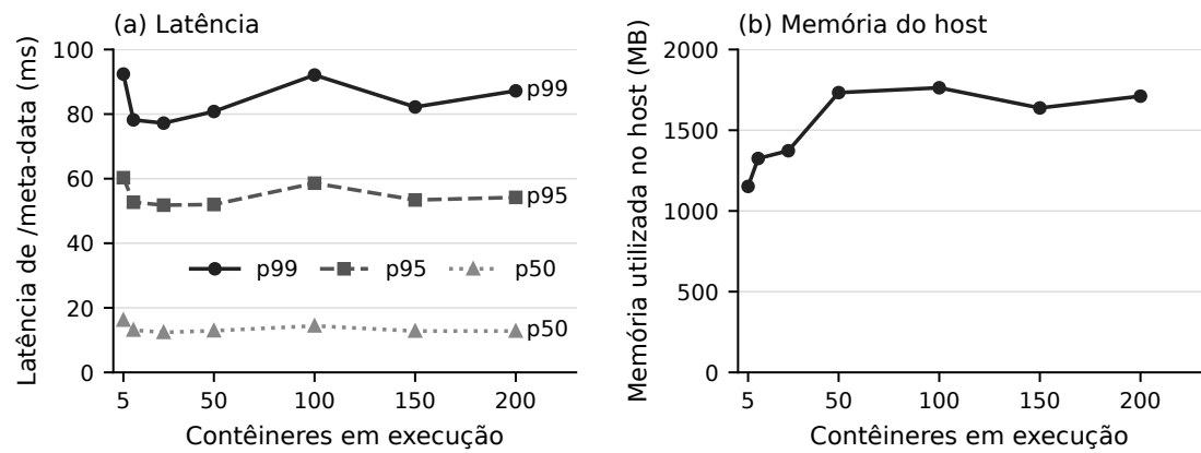
Figura 2. Escalabilidade em host único com contêineres de sistema: (a) latência de /meta-data nos percentis p50, p95 e p99 e (b) memória utilizada no host, por número de contêineres em execução. Uma execução de 5000 requisições (concorrência 50) por configuração; valores indicativos.
