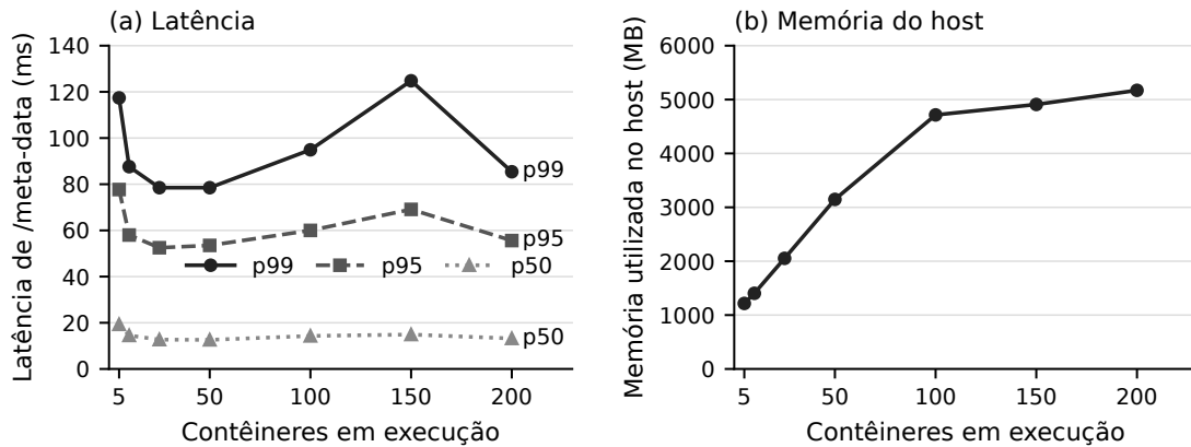
Figura 2. Escalabilidade em host único com contêineres de sistema: (a) latência de /meta-data nos percentis p50, p95 e p99 e (b) memória utilizada no host, por número de contêineres em execução. Uma execução de 5000 requisições (concorrência 50) por configuração; valores indicativos.
