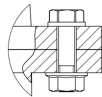
SZCZEGÓŁ C SKALA 1 : 1
