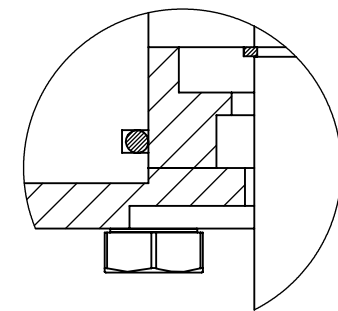
SZCZEGÓŁ B SKALA 1 : 1
