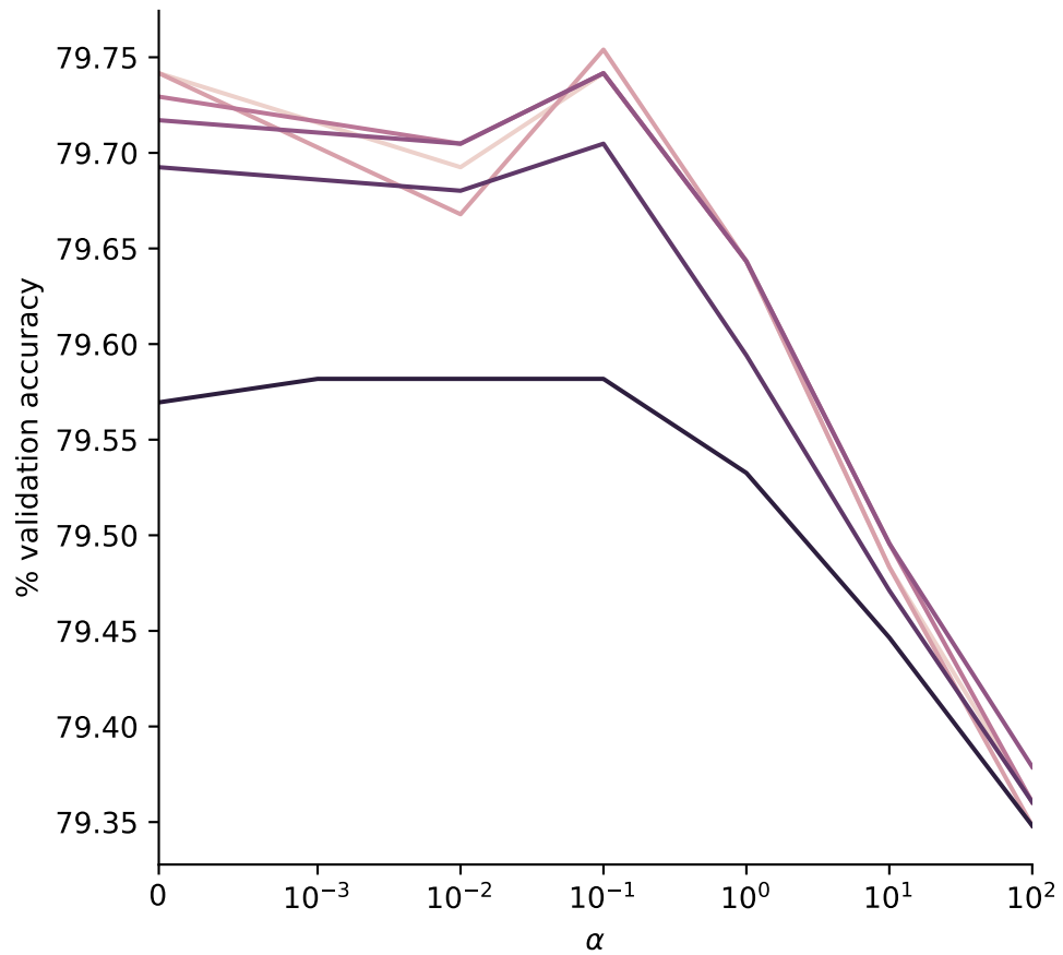
dataset = Cora
