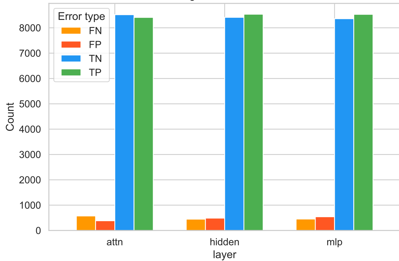
gemma-2-9b-it
