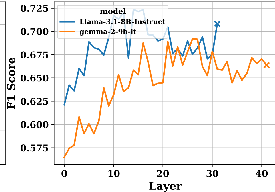
HaluEval
