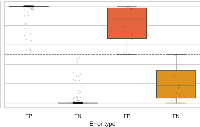
gemma-2-9b-it
