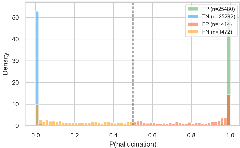
gemma-2-9b-it
