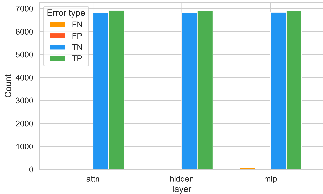
gemma-2-9b-it
