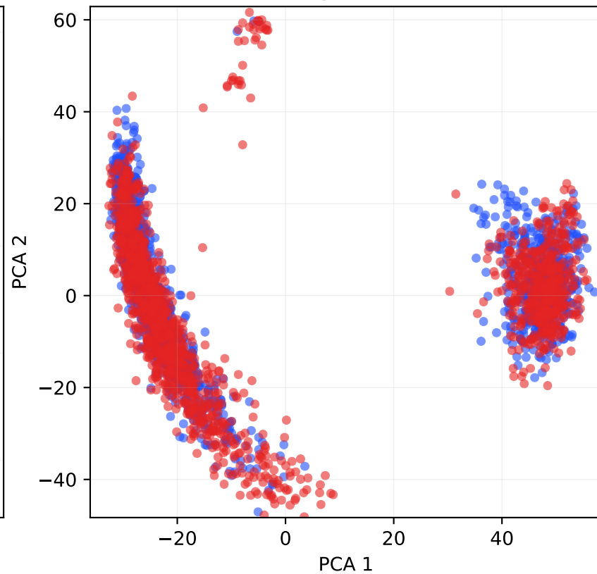
HaluEval (Layer 19)
