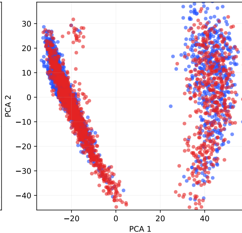
HaluEval (Layer 23)
