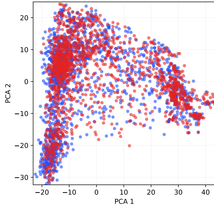
HaluEval (Layer 14)
