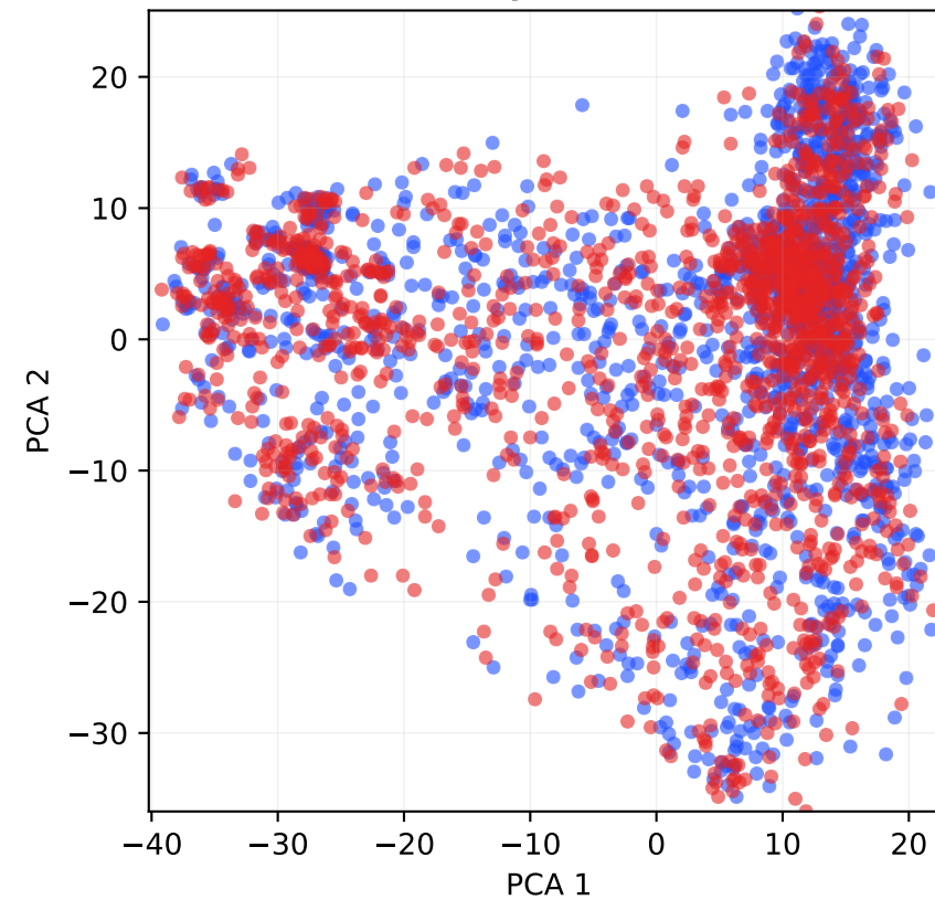
HaluEval (Layer 13)
