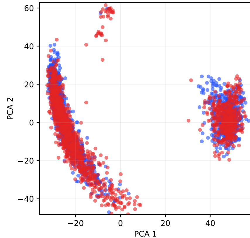
HaluEval (Layer 19)
