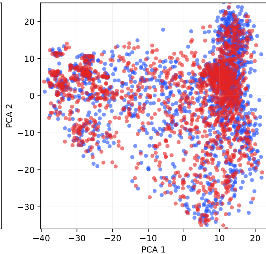
HaluEval (Layer 13)
