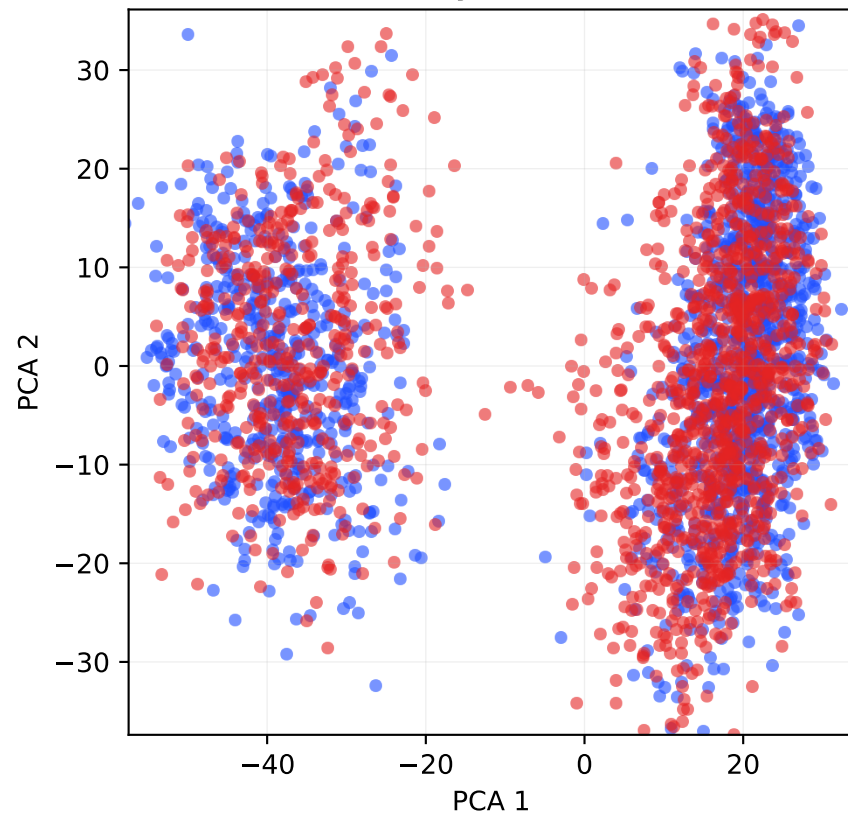
HaluEval (Layer 21)
