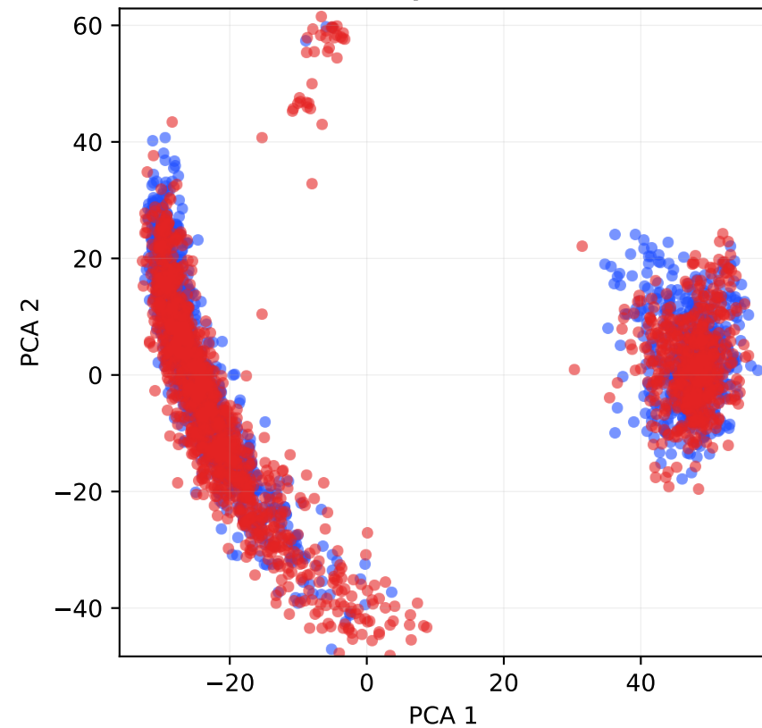
HaluEval (Layer 19)
