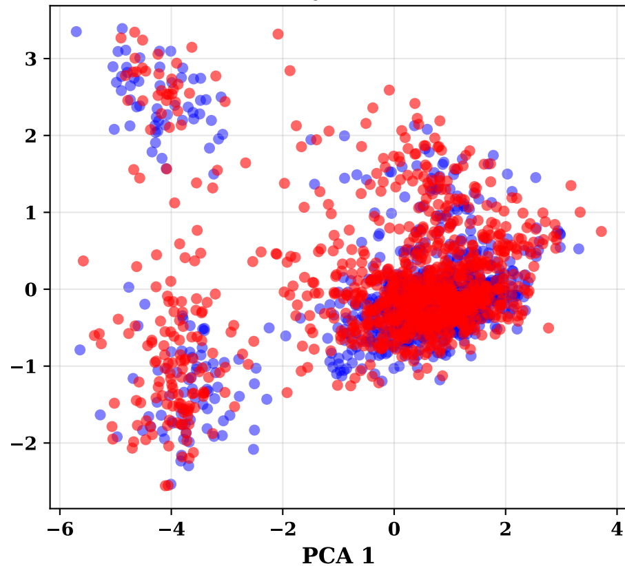
HaluEval (Layer 21)
