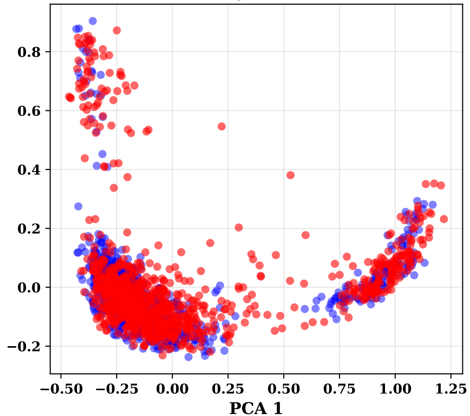
HaluEval (Layer 23)
