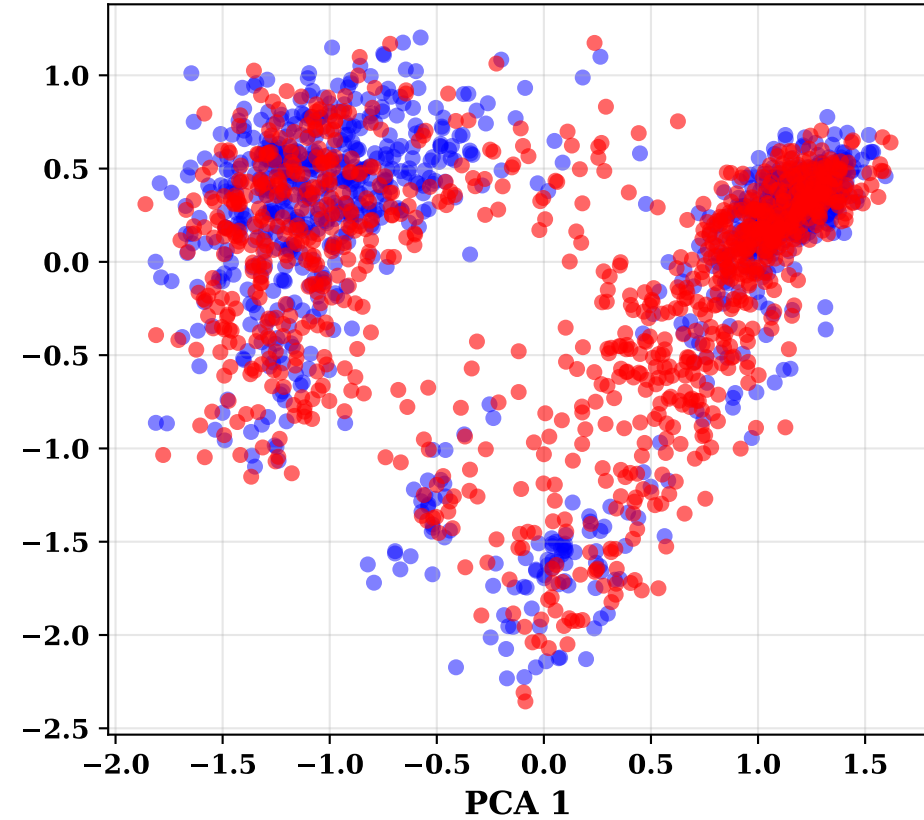
HaluEval (Layer 14)
