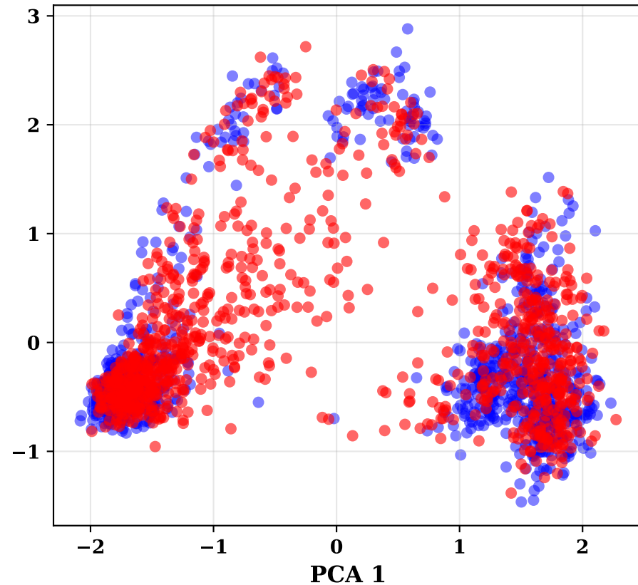
HaluEval (Layer 13)
