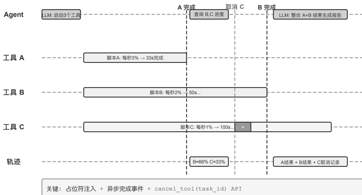
图 4-6 实验 4-5 异步 Agent 打断与恢复
