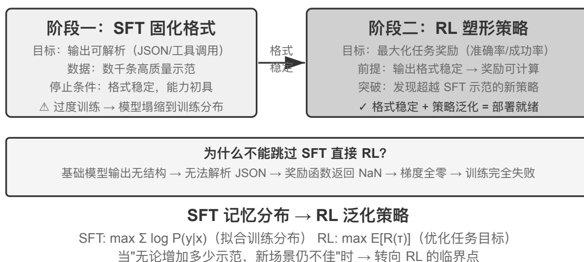
图 7-11 SFT → RL 两阶段训练流程
