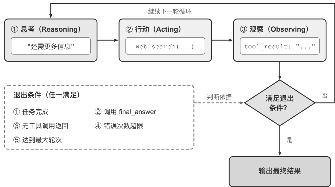
图 1-5 自主 Agent 的执行循环
