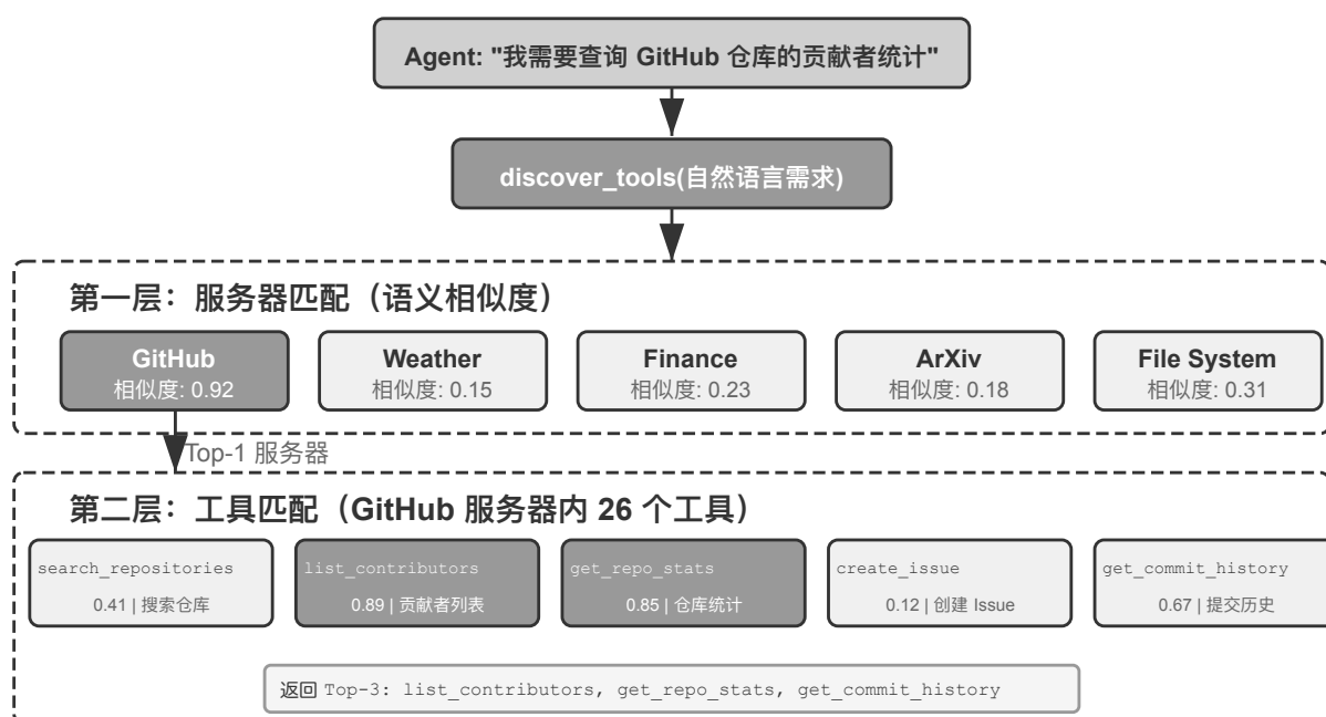
图 4-7 层次化工具匹配（服务器级 → 工具级两层语义搜索）
