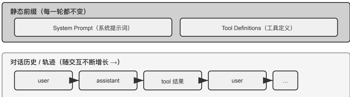
“静态前缀 + 轨迹”结构：前缀不能动（利于 KV Cache），轨迹可压缩
