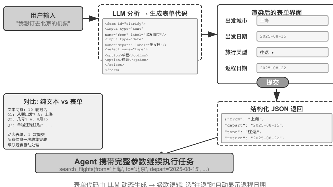
图 5-8 动态表单生成流程
