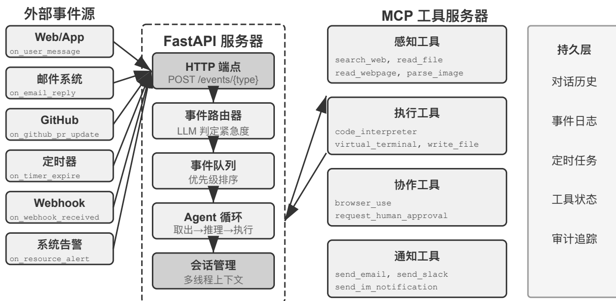
图 4-4 实验 4-4 事件驱动 Agent 架构
