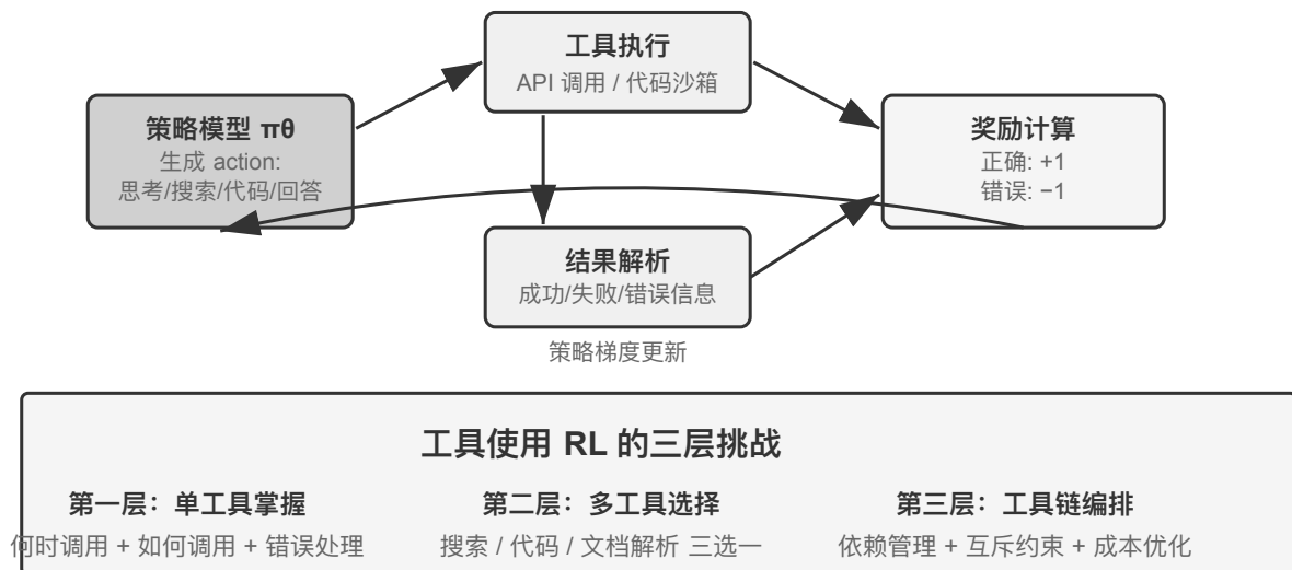
图 8-16 工具调用 RL 奖励循环
