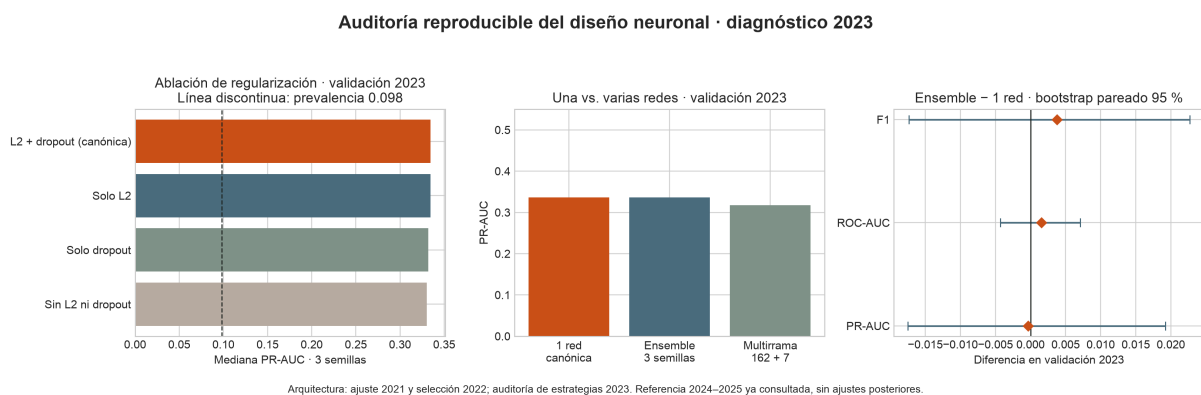
Figura 18: Auditoría 2023 de regularización y número de redes. El eje derecho muestra diferencias pareadas del ensemble respecto de la red única; los intervalos incluyen cero.
