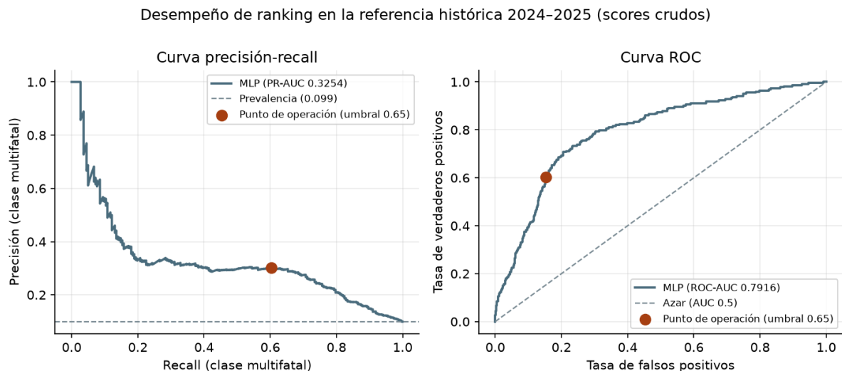
Figura 20: Curvas precisión-recall y ROC sobre los scores crudos de la referencia histórica. El punto de operación corresponde al umbral 0.65 fijado en 2023: recall 0.604 con precisión 0.302, sobre una tasa de falsos positivos de 0.154.
