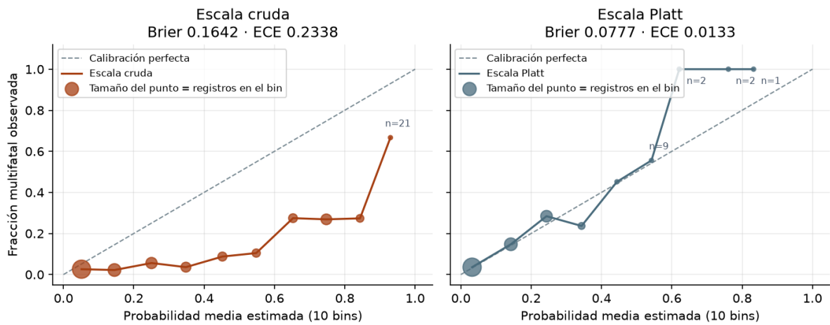
Figura 21: Diagrama de confiabilidad por decil de probabilidad. El tamaño del punto es proporcional al número de registros del bin; se anota n cuando el bin reúne 25 registros o menos.
