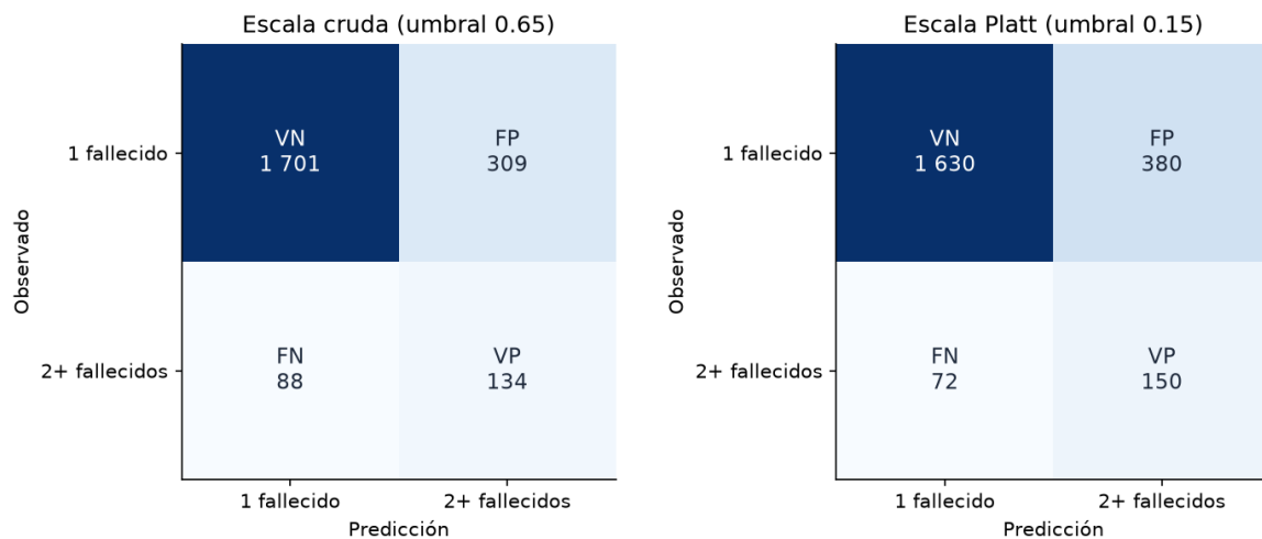
Figura 22: Matrices de confusión en ambas escalas. El umbral calibrado convierte 16 falsos negativos en verdaderos positivos (de 88 a 72) al precio de 71 falsas alertas adicionales (de 309 a 380): el desplazamiento de umbral redistribuye el error, no lo elimina.
