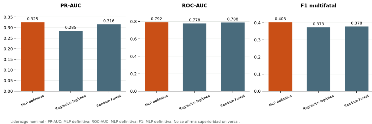
Figura 23: Comparación descriptiva en la referencia histórica 2024–2025 sobre scores crudos. El liderazgo nominal no equivale a superioridad universal.
