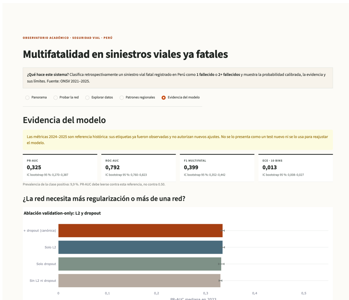
Figura 27: Sección Evidencia del modelo . Cada métrica aparece con su intervalo de confianza y la prevalencia se declara junto a PR-AUC, de modo que la cifra no pueda leerse contra 0.50 por descuido.
