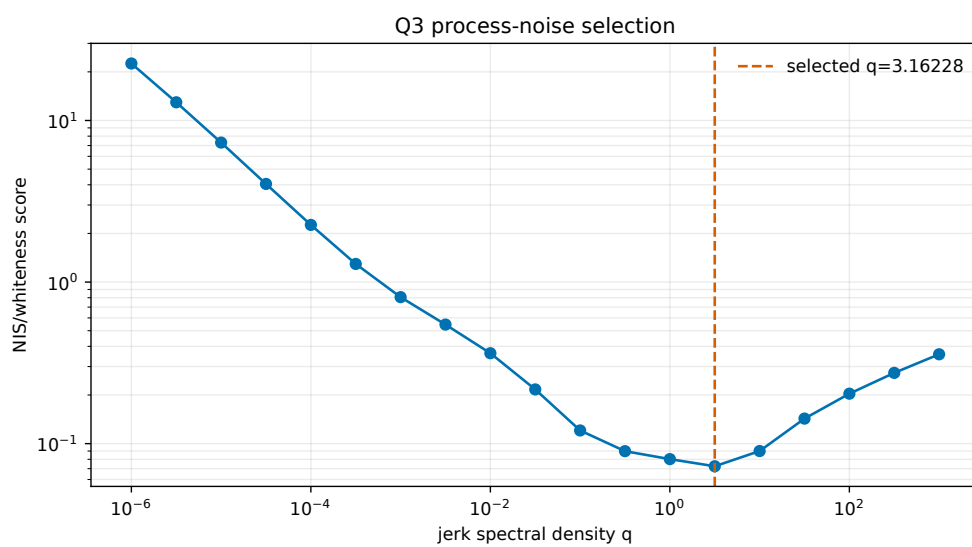
图 14 问题三过程噪声参数选择
