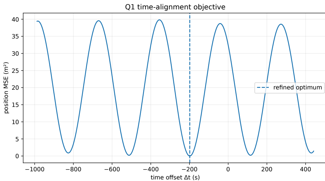
图 1 问题一全域时间偏差目标函数扫描
