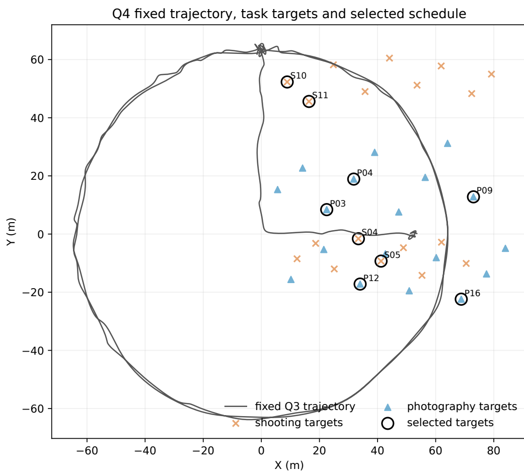
图 12 问题四轨迹、目标点与所选任务
