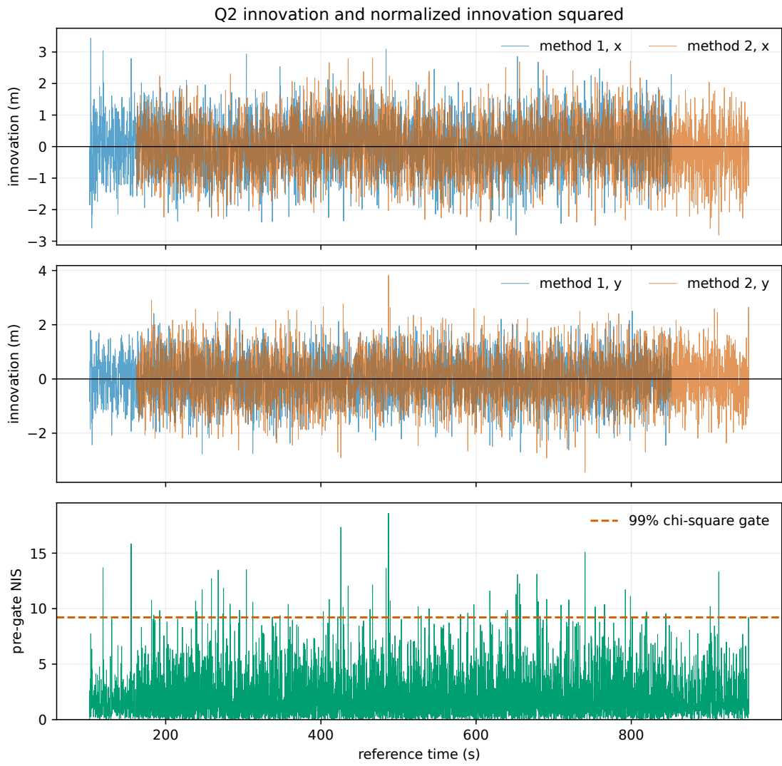
图 7 问题二白化创新与预检验 NIS 诊断
