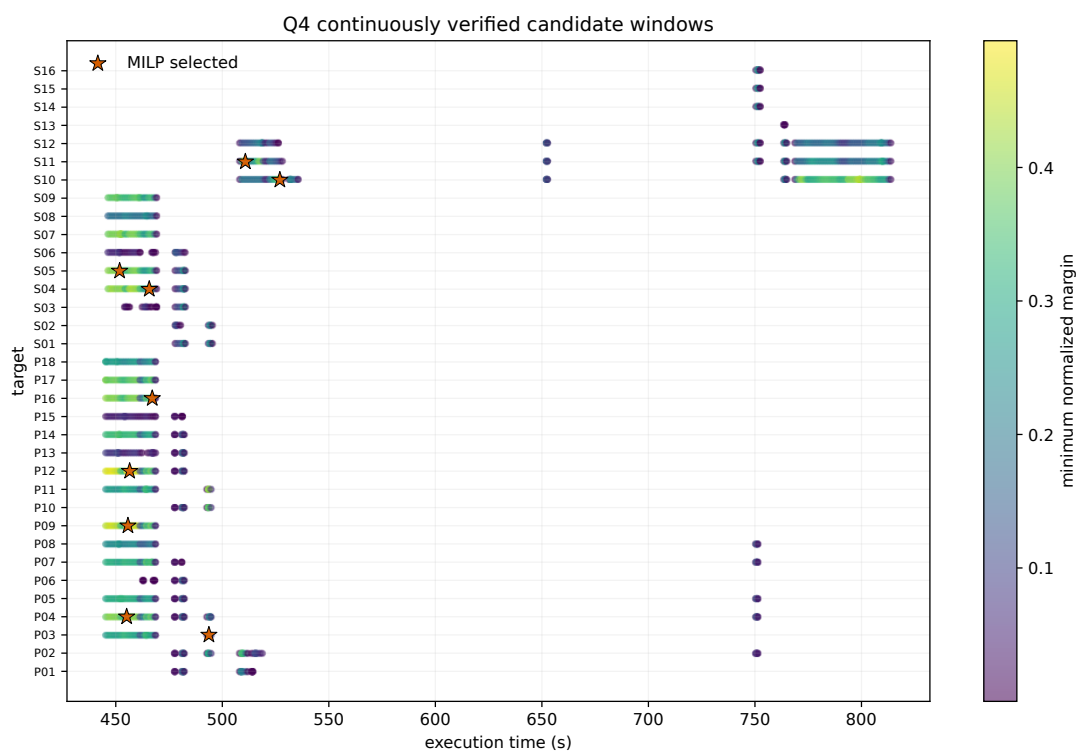
图 13 问题四连续复核后的候选任务分布
