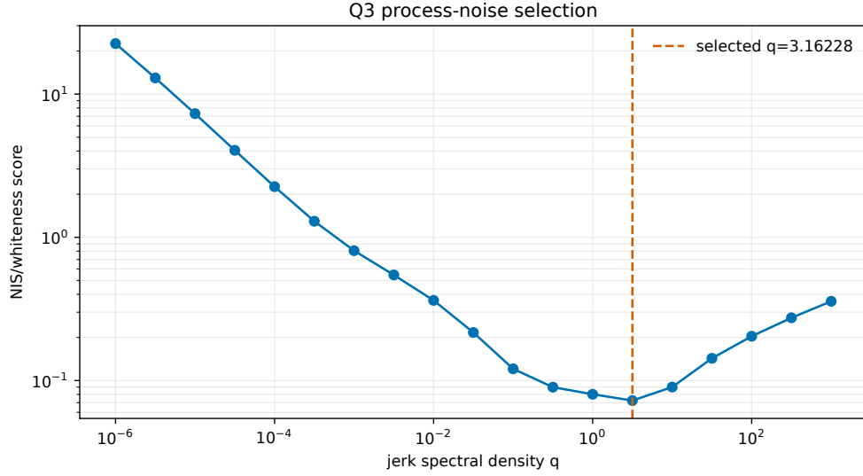
图 11 问题三过程噪声参数选择
