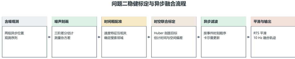
图 5 问题二稳健标定与异步融合流程
