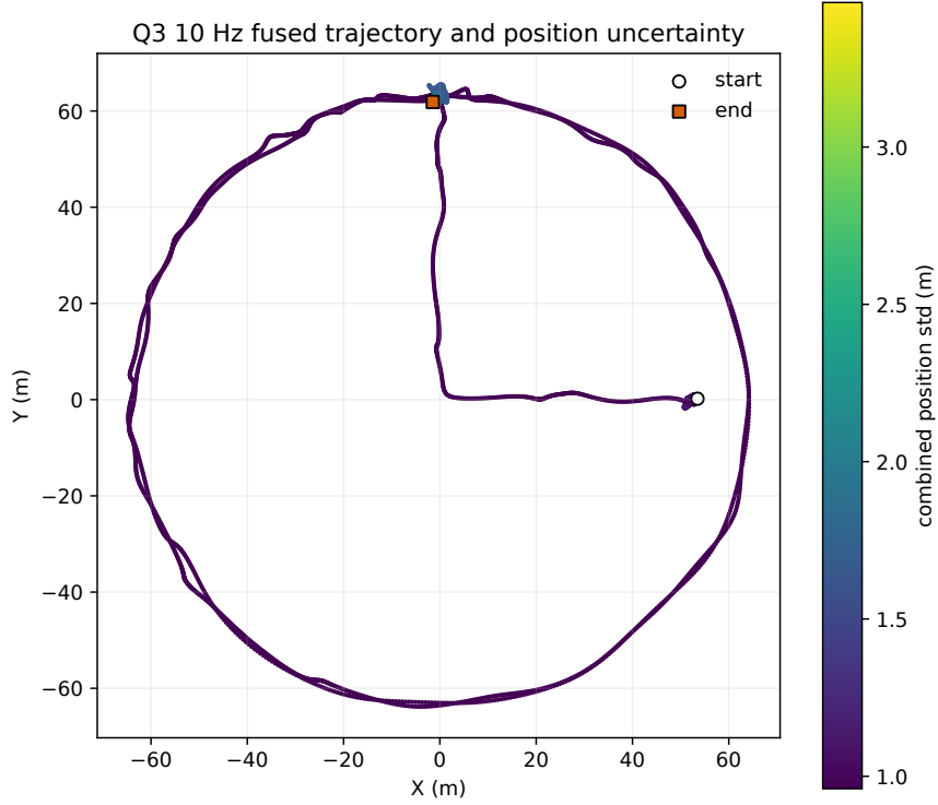
图 13 问题三 10 Hz 融合轨迹及模型内位置标准差
