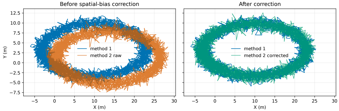
图 7 问题二时空校正前后的两设备二维位置
