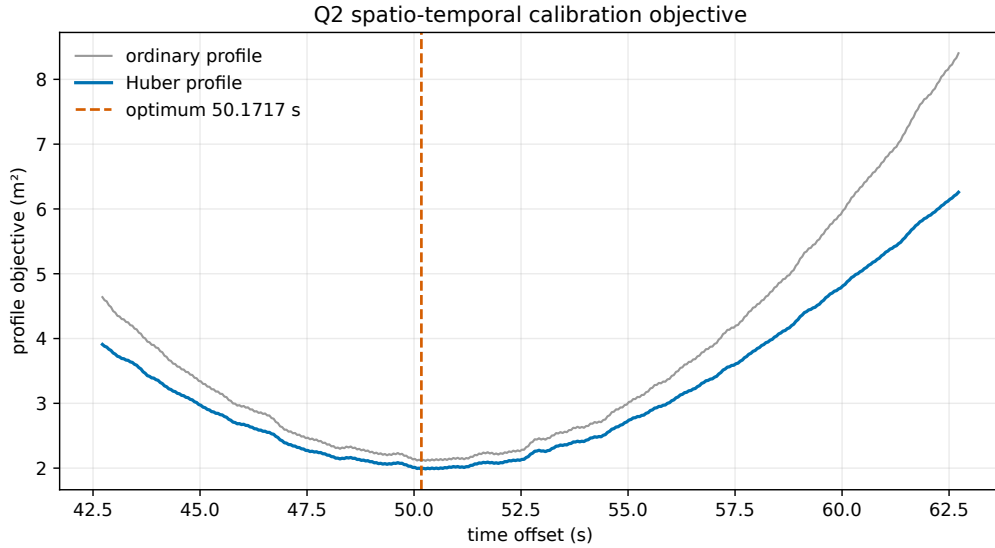
图 6 问题二时空标定目标函数剖面
