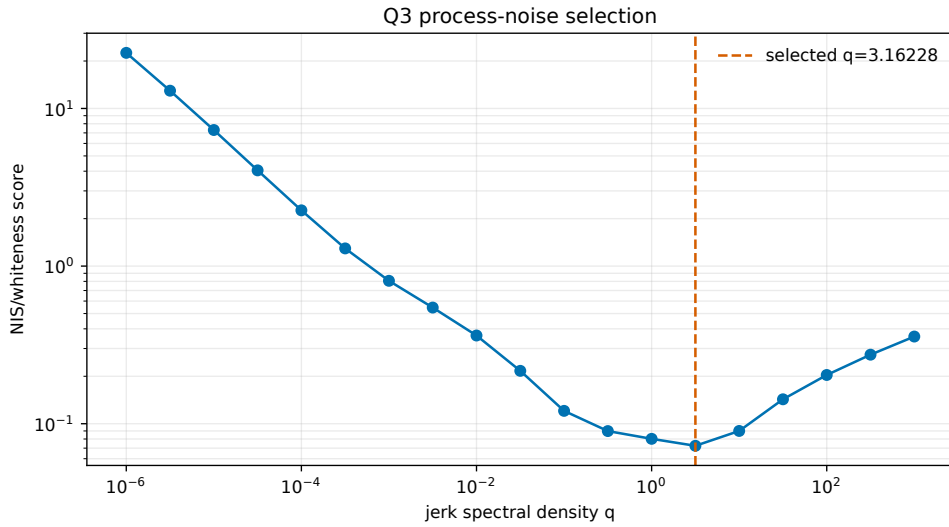
图 12 问题三基于门控前创新统计的过程噪声选择
