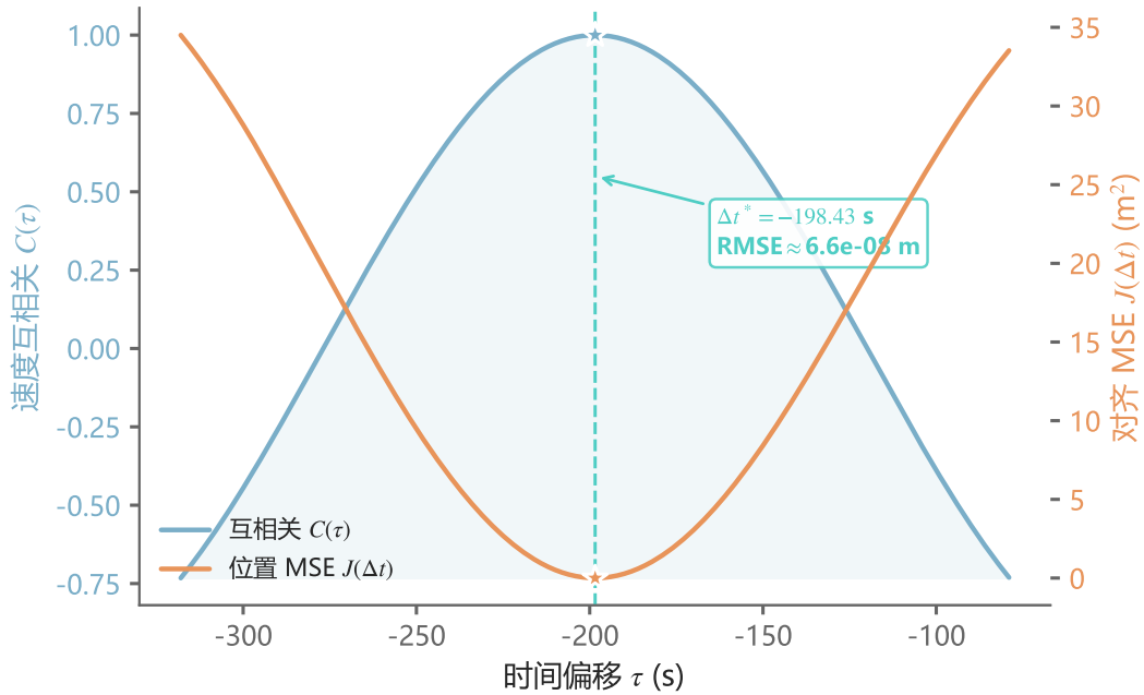
图 2 模型一速度互相关与时间对齐目标函数
