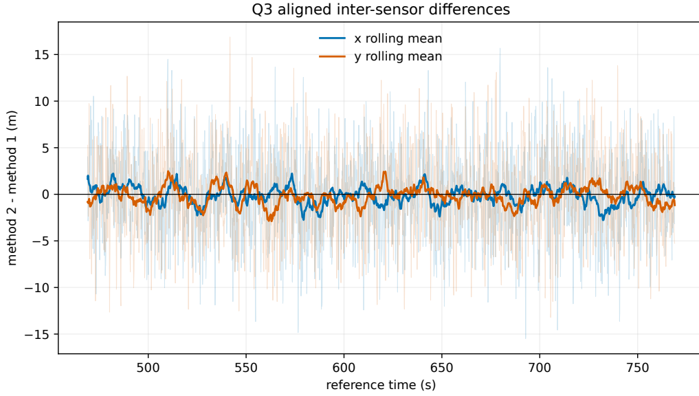
图 11 问题三时间配准后的两坐标相对残差时序
