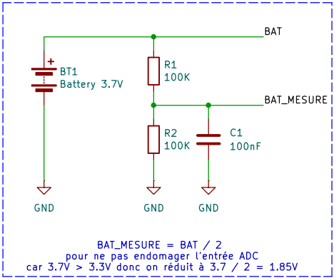
Batterie
