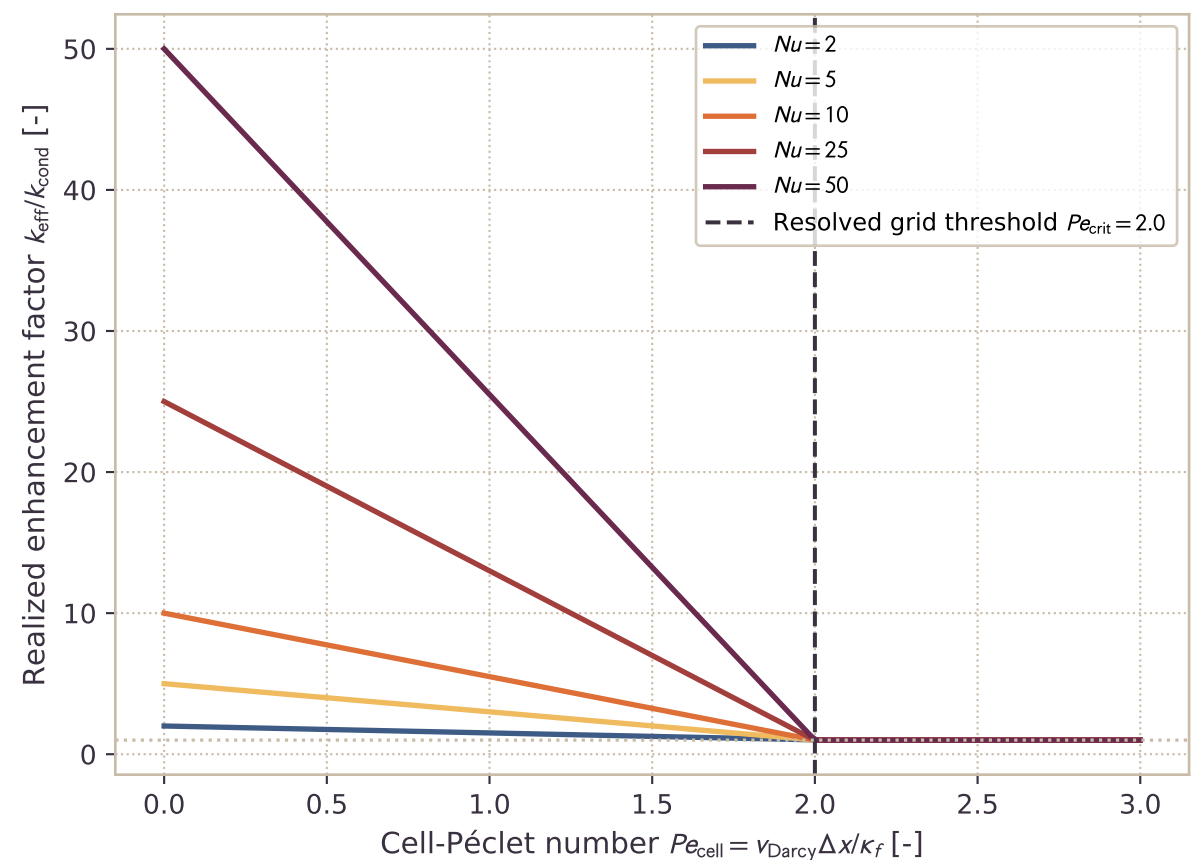
(d) Grid-Resolution Damping (Prevent Double Counting)
