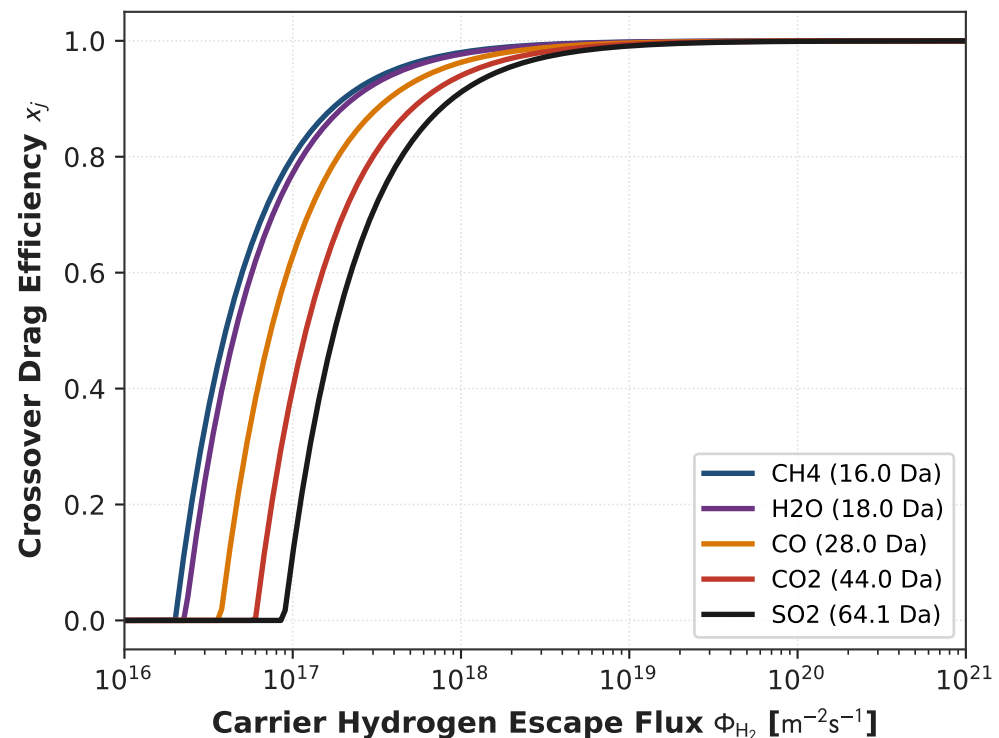
(d) Zahnle-Kasting Hydrodynamic Crossover Drag
