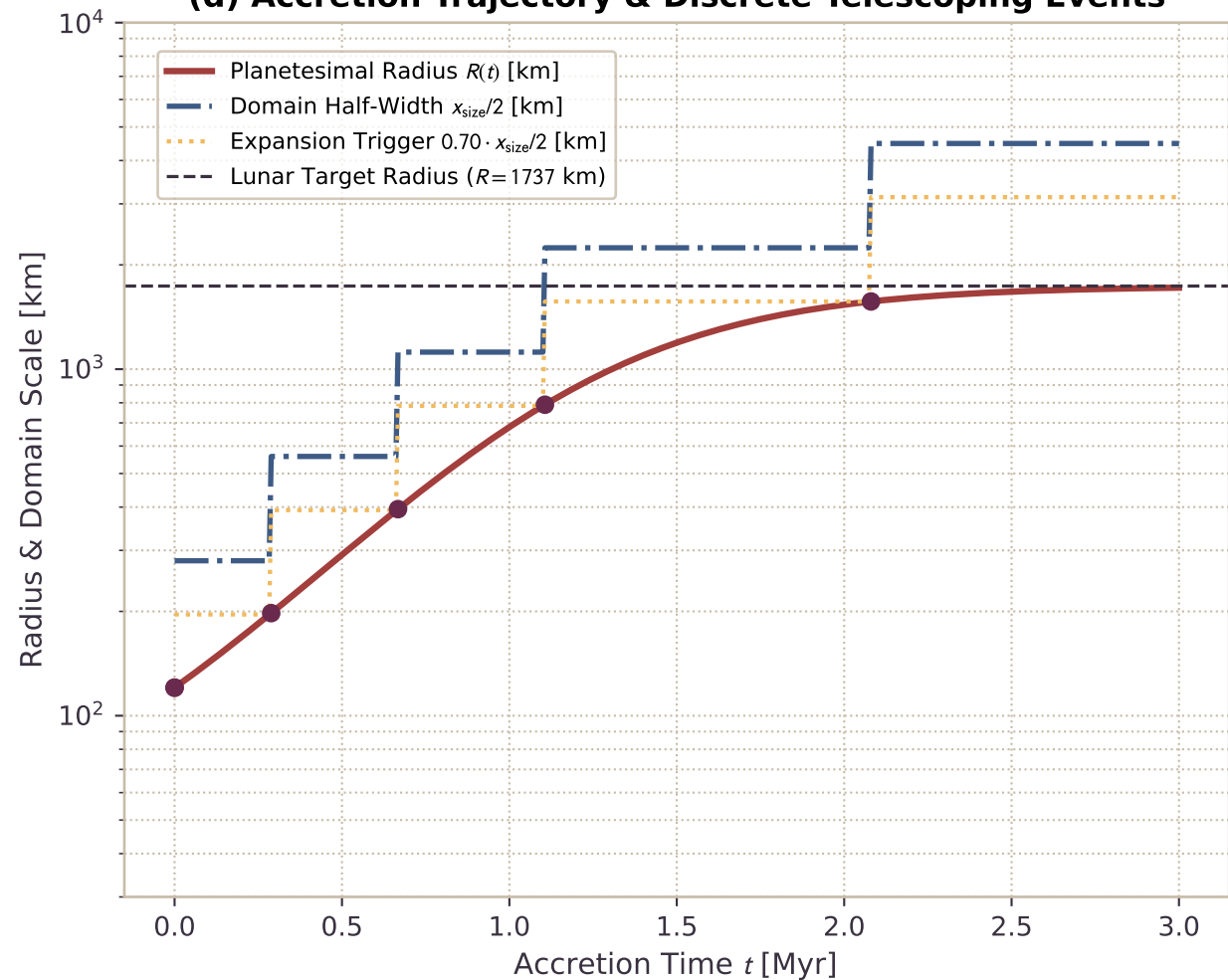
(d) Accretion Trajectory & Discrete Telescoping Events
