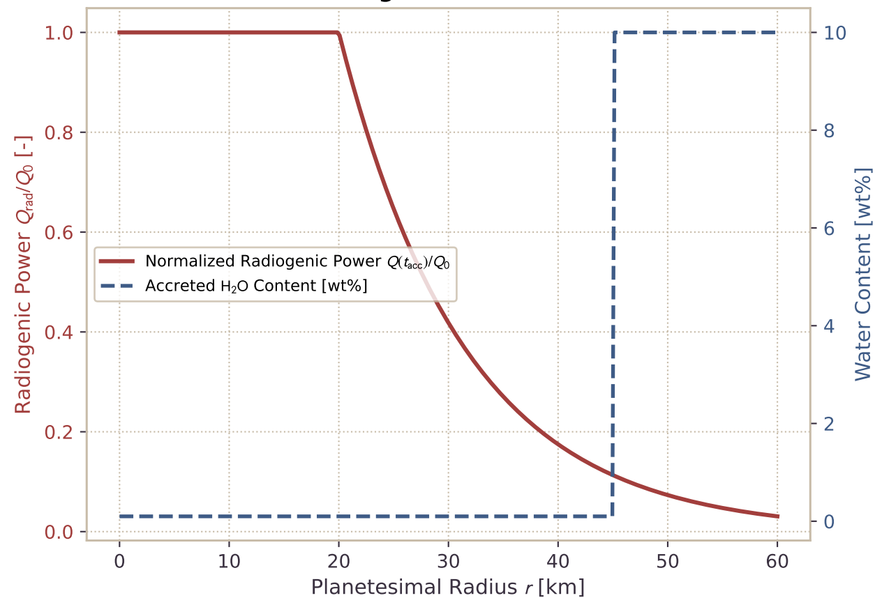
(d) Onion-Shell Radiogenic Clock & Snowline Volatiles
